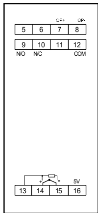
D71接线图
