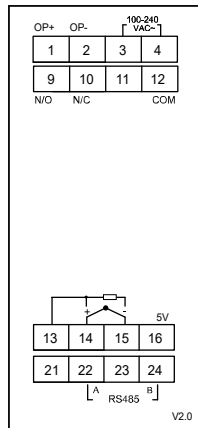
E71接线图
